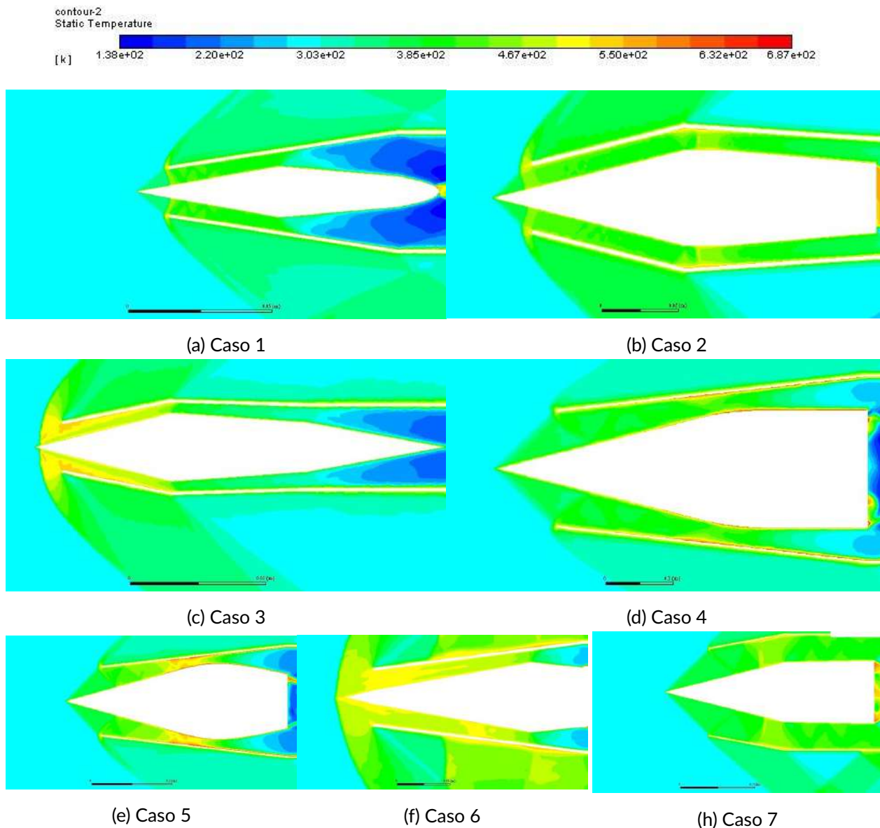
FIG. 10 Distribución de la temperatura estática en el difusor de entrada.
