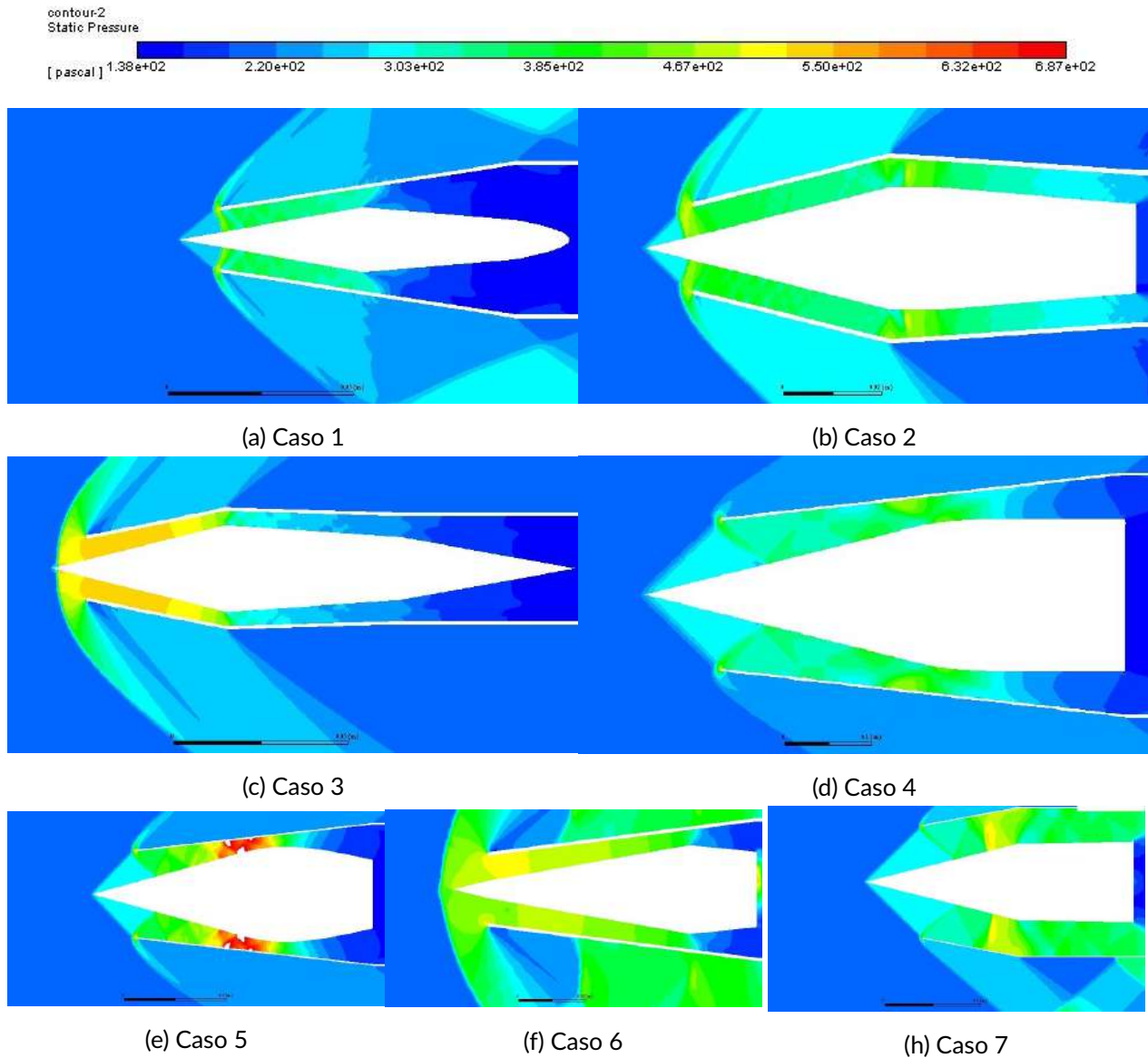
FIG. 9 Distribución de la presión estática en el difusor de entrada.
