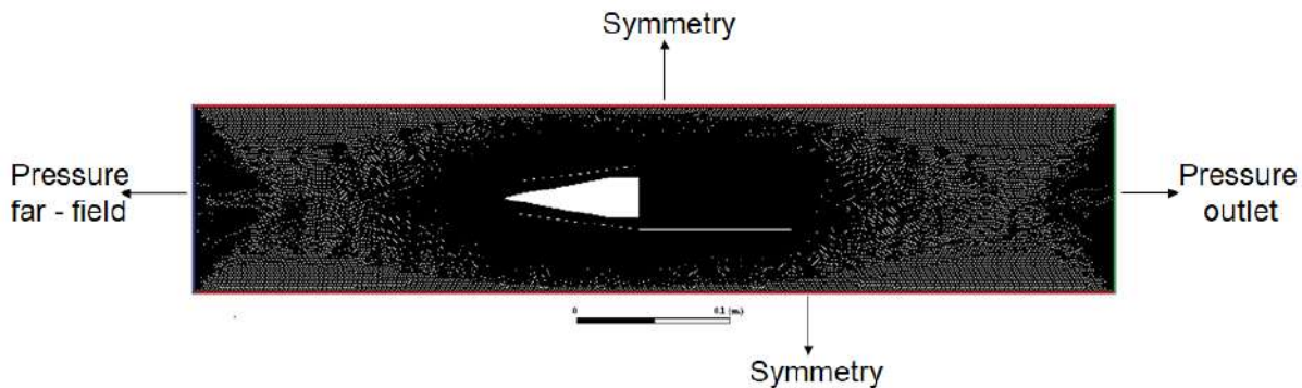
FIG. 6 Condiciones de contorno.
