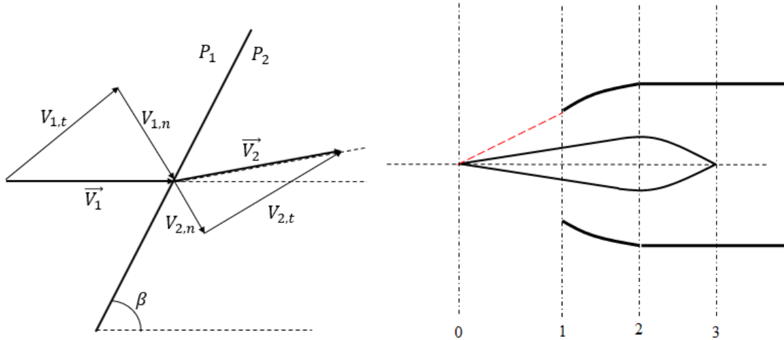
FIG. 3 Choque oblicuo en una cuña.
